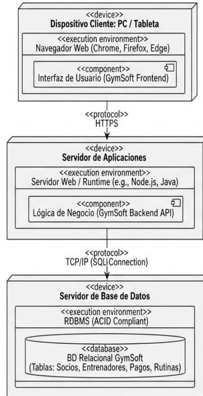
Diagrama de Despliegue - Sistema GymSoft
